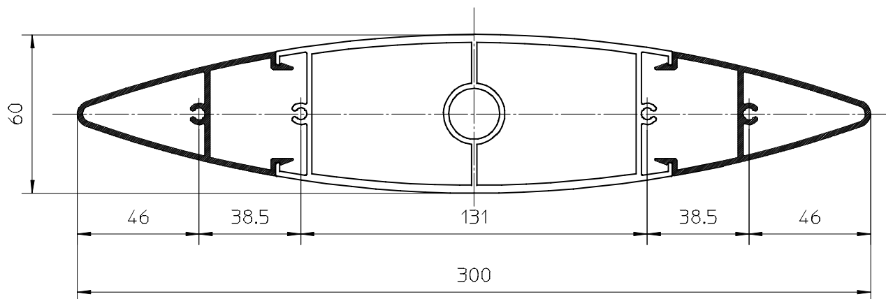
Perfil F.016.014
